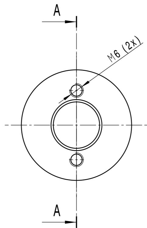
Front view Scale: 1:1
