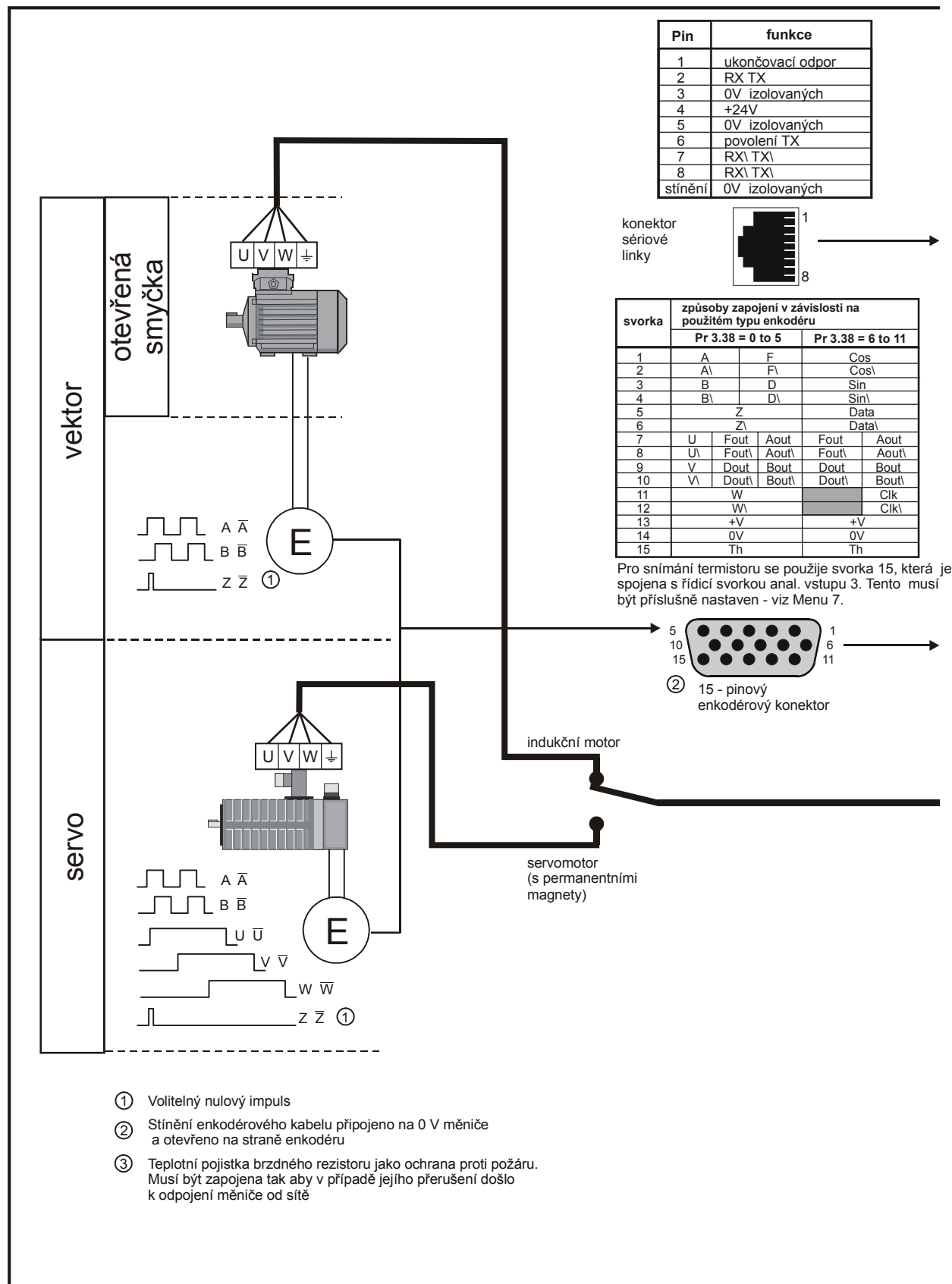
Obr. 7-1: Minimální zapojení pro všechny kategorie
