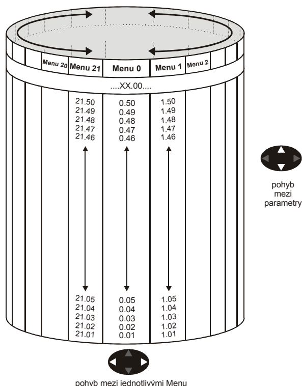
Obr. 4-2: Struktura parametrů
