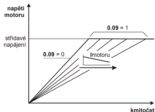
Obr. 6-1: Pevná a dynamická charakteristika U/f
