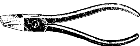
A DRÁT, širokočelistné DRAHTZANGEN mit breitem Maul délka - Länge mm: 160 185 210 jemné, černé 1 kus } Kč 14.35 15.80 18.20 schwarz 1 Stk
