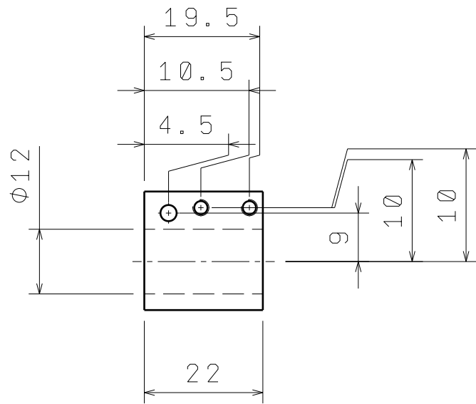
Right view Scale: 1:1
