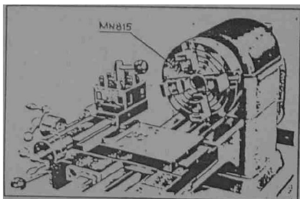
MN 815 – upínací deska \varnothing 150 mm se čtyřmi otočnými čelistmi
