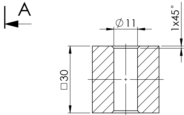
ŘEZ A-A MĚŘÍTKO 1 : 1
